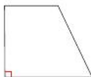
直角梯形
