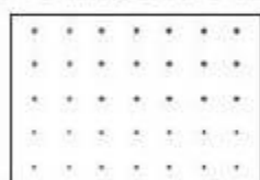
等腰三角形
